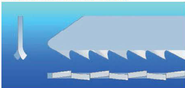
Dientes fresados corte libre triscado
