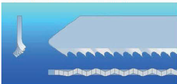
Dientes fresados corte libre ondulado
