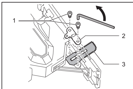
▶ 1. Parafusos passantes 2. Porta-lâmina 3. Lâmina
