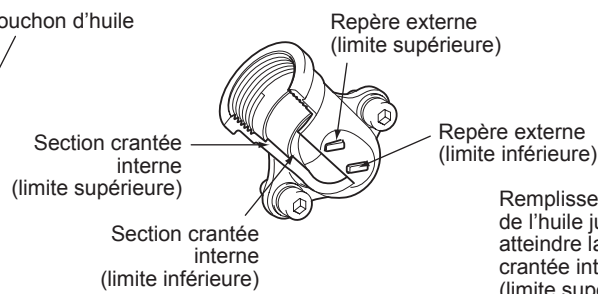
Fig. 2 Tuyau d'huile
