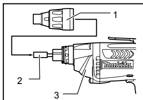
1. Bague de retenue 2. Embout à douille magnétique 3. Carter d'engrenage
