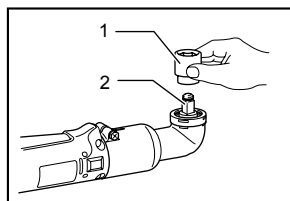
1. Douille 2. Enclume
