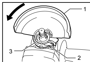
1. Carter de meule 2. Vis 3. Cage de roulement
