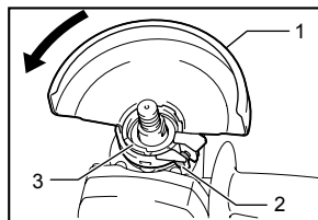
1. Protector (guarda) de disco 2. Tornillo 3. Caja de rodamientos
